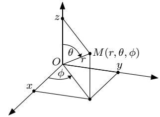
FIG. 5.5 – Coordonnées sphériques.
