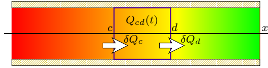
FIG. 3.1 – Cylindre chargé.
