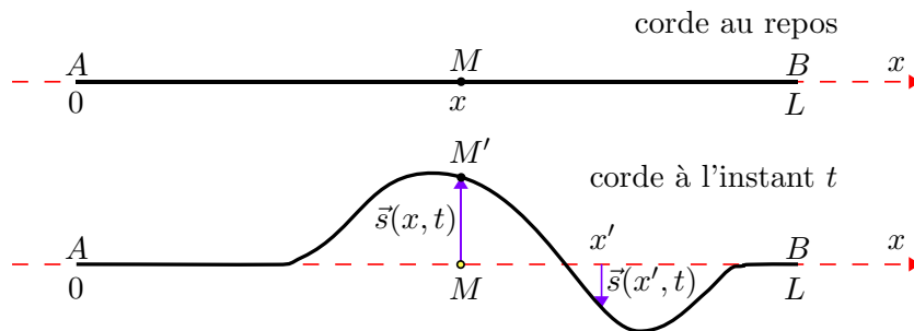
FIG. 1.1 – Corde vibrante.
