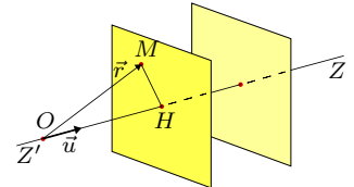
FIG. 5.1 – Plans d'ondes.
